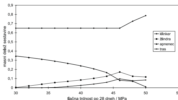
Slika 1: Optimalne sestave mešanih portlandskih cementov za različne trdnosti. Izračun velja za najdaljši čas mletja (25 min v laboratorijskem mlinu) in za sestave brez aditiva CBA 1110. Vsi cementi vsebujejo poleg teh komponent še 5% gipsa
